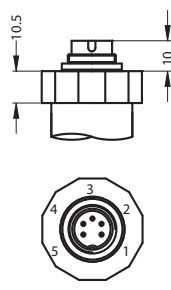
Binder 723 (IP 67)
