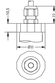
Кабельный ввод (IP 67) 1,2
