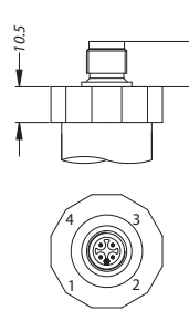
M12x1 (4 конт.) (IP 67)
