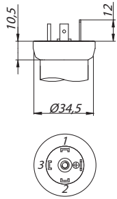
DIN 43650 (IP 65/IP 67)
