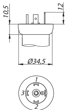
DIN 43650
