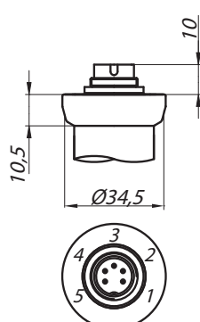
Binder 723 (5-конт.)
