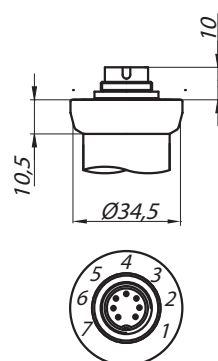
Binder 723 (7-конт.)
