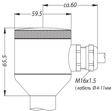
Корпус для полевых условий
