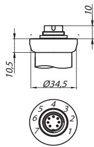
Binder 723 (7-конт.)
