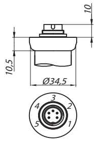
Binder 723 (5-конт.)
