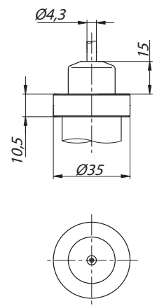
Кабельный ввод без трубки компенсации атмосферного давления
