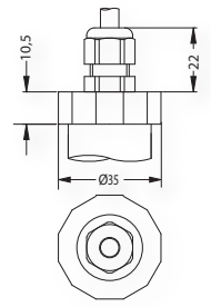
Кабельный ввод
