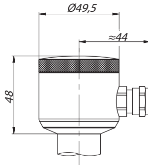
Компактный полевой корпус
