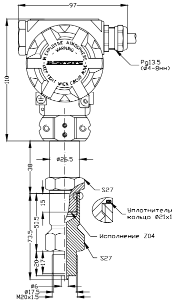
M20x1.5 (Z04) с адаптером – код G04
