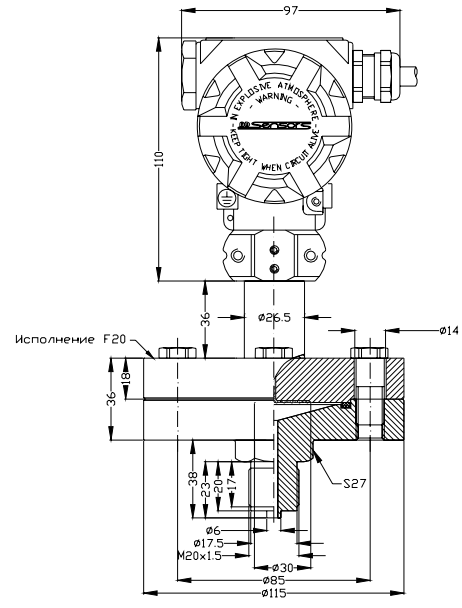
Фланцевое исполнение (F20) с адаптером – код G20
