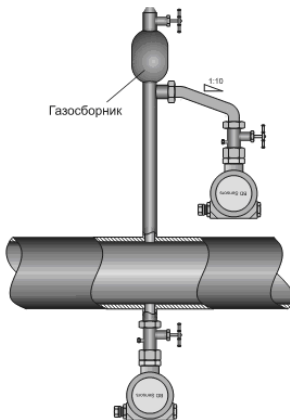
Рисунок 2. Монтаж датчика для измерения давления жидкости.
