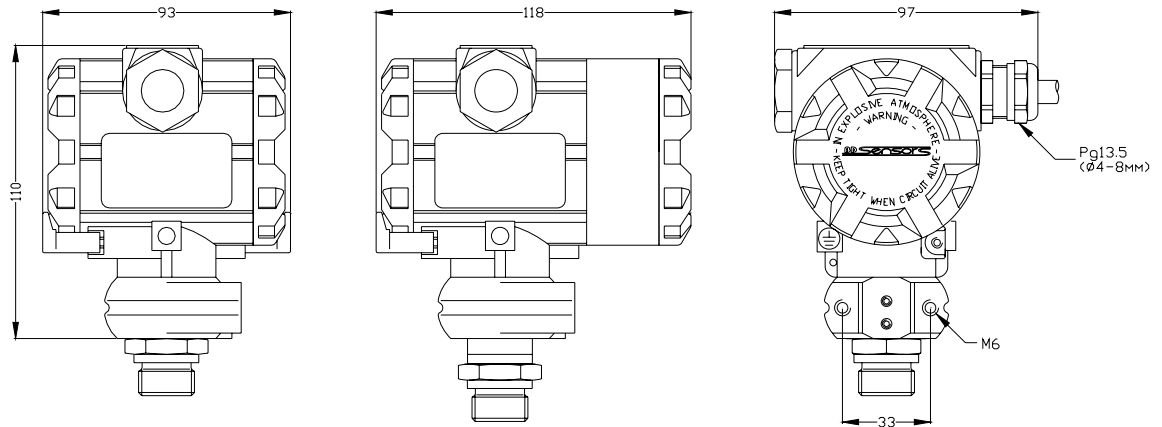
Рисунок Б.1 – Датчик НМР 331 без разделителя.
