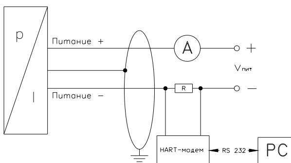
2-х пров. / HART
